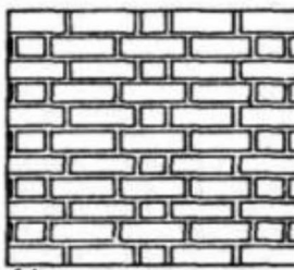
фламандская изгородь
