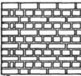
Английская крестовая (перевязка – крест св. Андрея)
