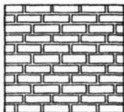
1/3 однорядная перевязка
