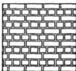
Английская перевязка
