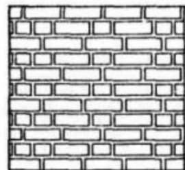
фламандская крестовая
